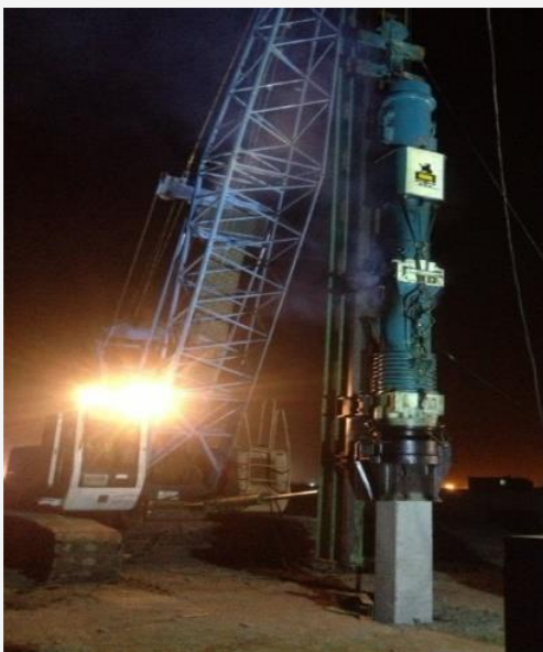
STARKE HD30 DIESEL-HAMMER
